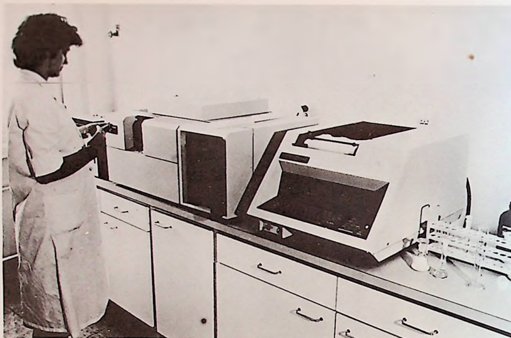
Plinski kromotograf PE-Sigma 1 B – za određivanje ostatka pesticida i organskih otapala u živežnim namirnicama, vodi i tlu.
