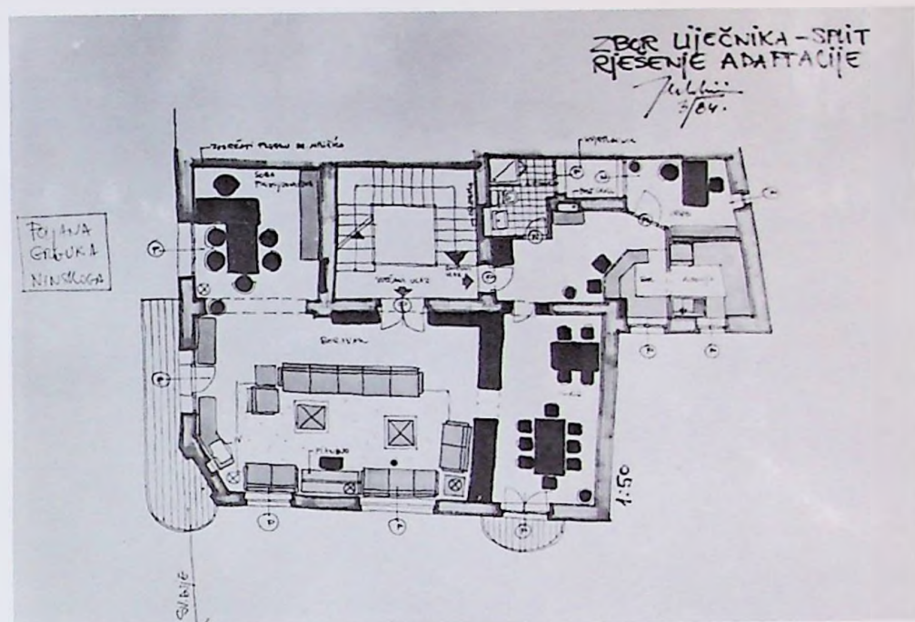
Tlocrt nove adaptacije prostorija Zbora u Splitu (ing. Jerko Rošin).
